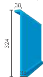
Sole Bar (ICF)
